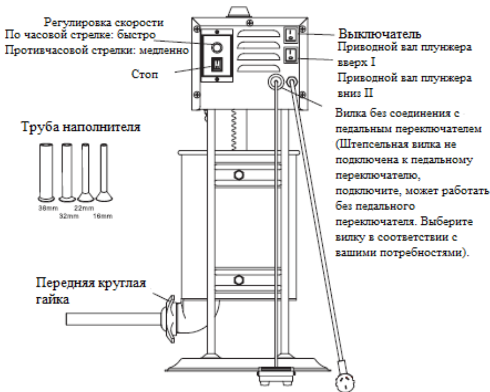
Рис2. Основные механизмы.
